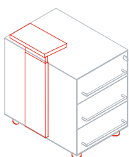
Supporto per cassettera portante (Graphis) 1BA1531: L 13 P 26 H 66
