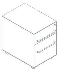
Cassettiera con 1 cassetto e 1 classificatore 1BA6012: L 40 P 56 H 56
